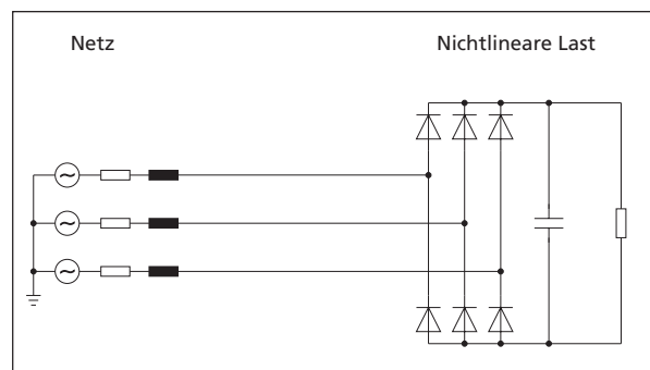
Abbildung 1: Ungesteuerter Diodengleichrichter
